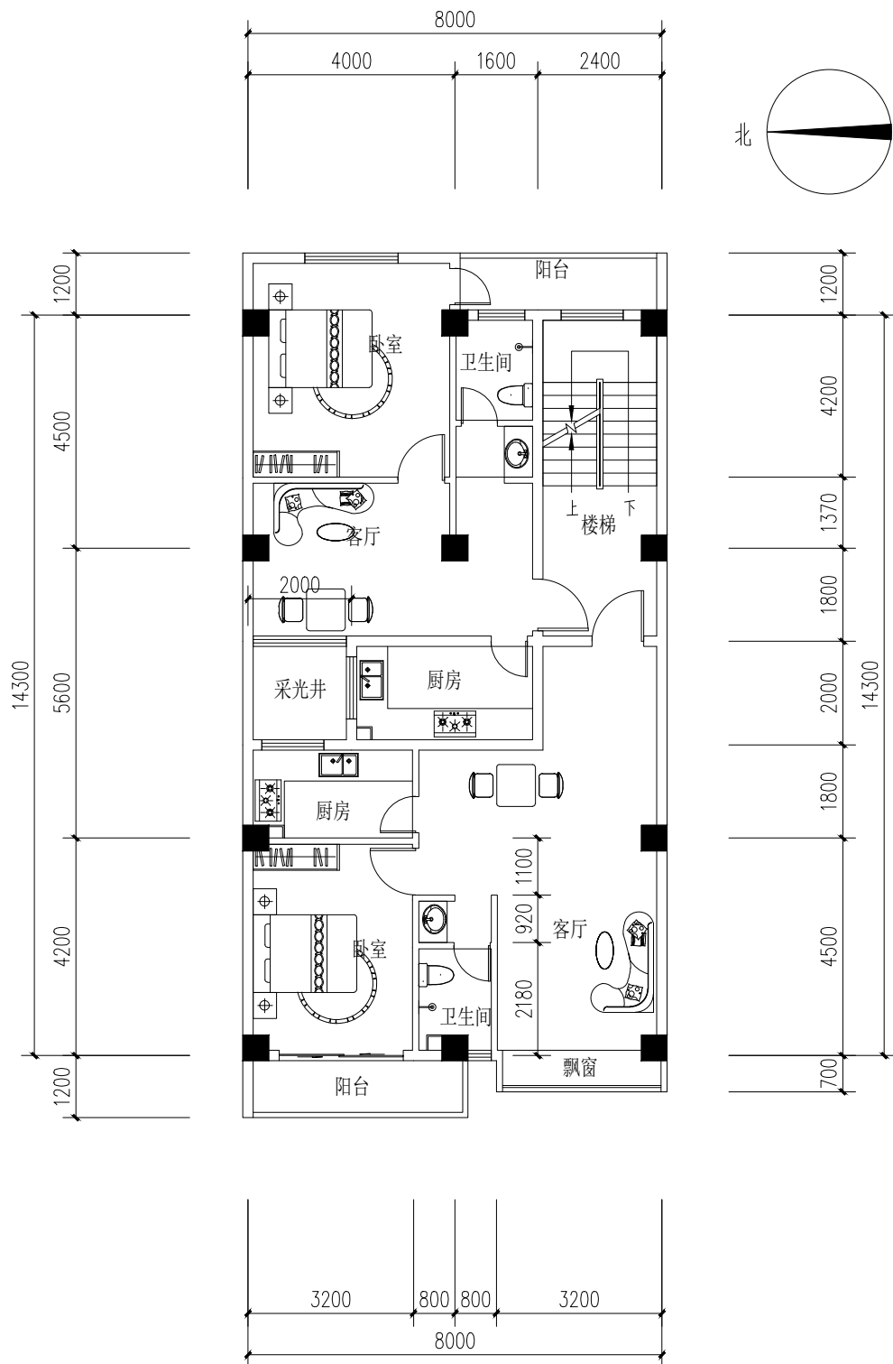
五、六层平面布局图 1 : 1 0 0
