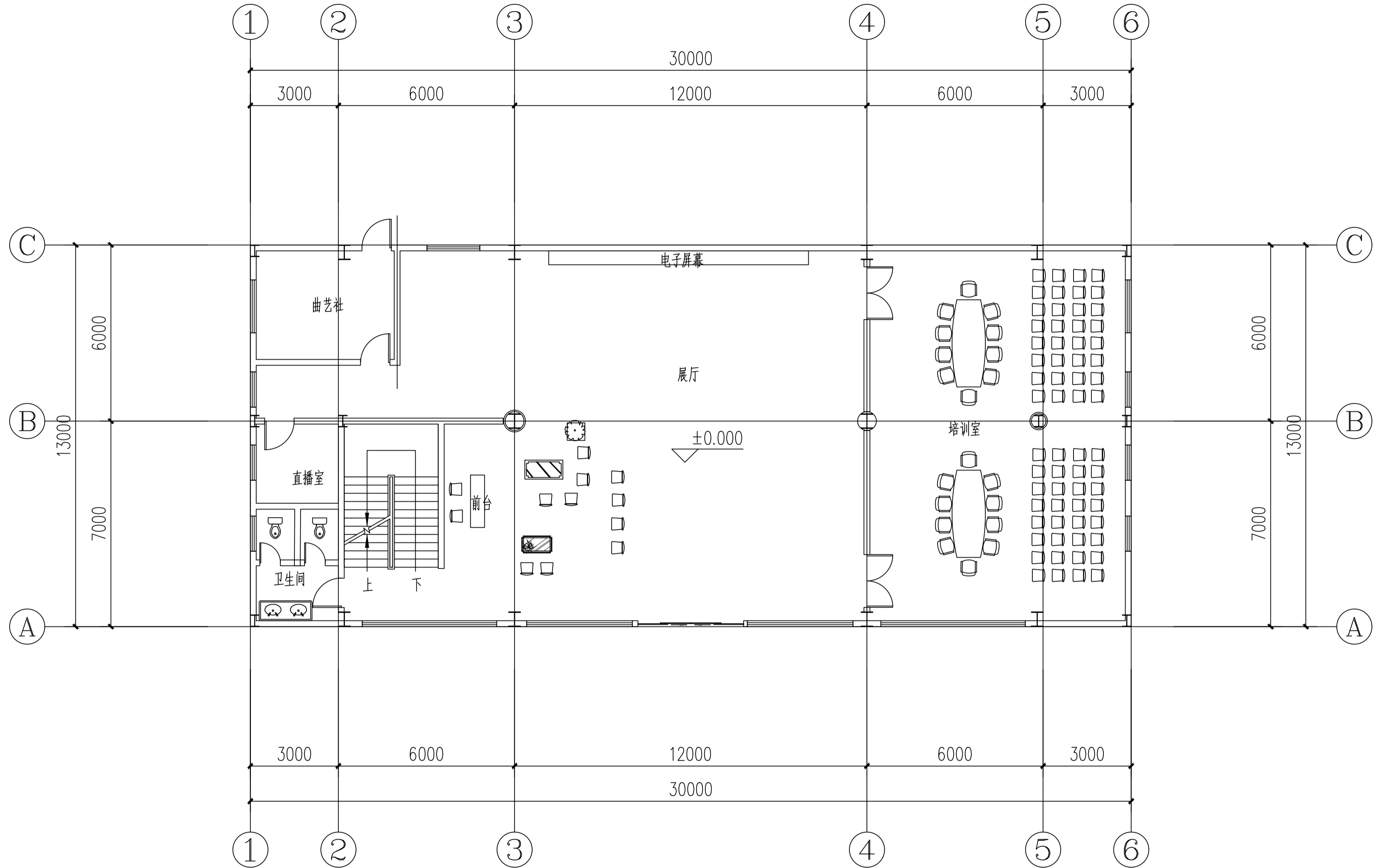
一层平面图 1:150
