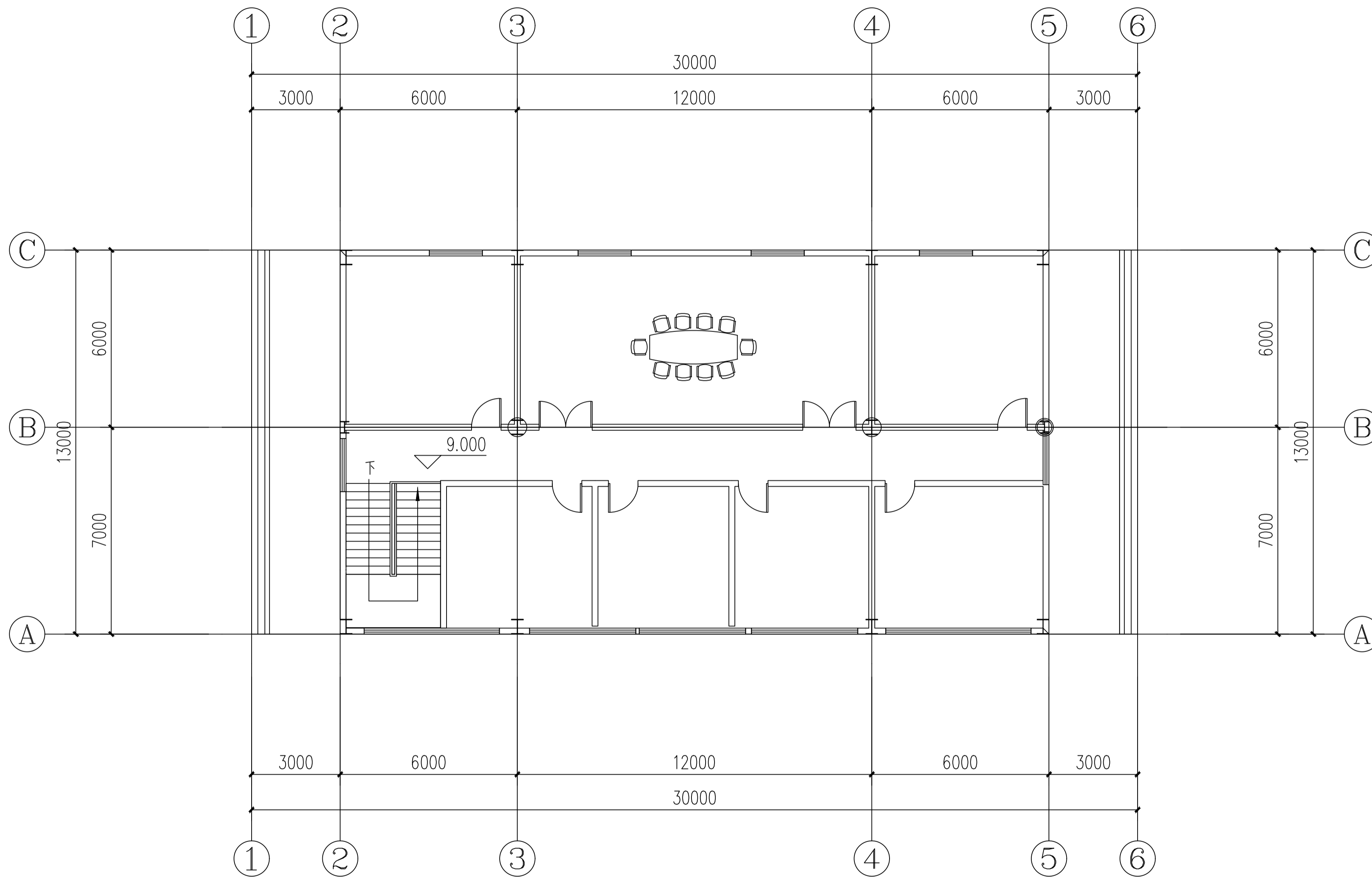
三层平面图 1:150
