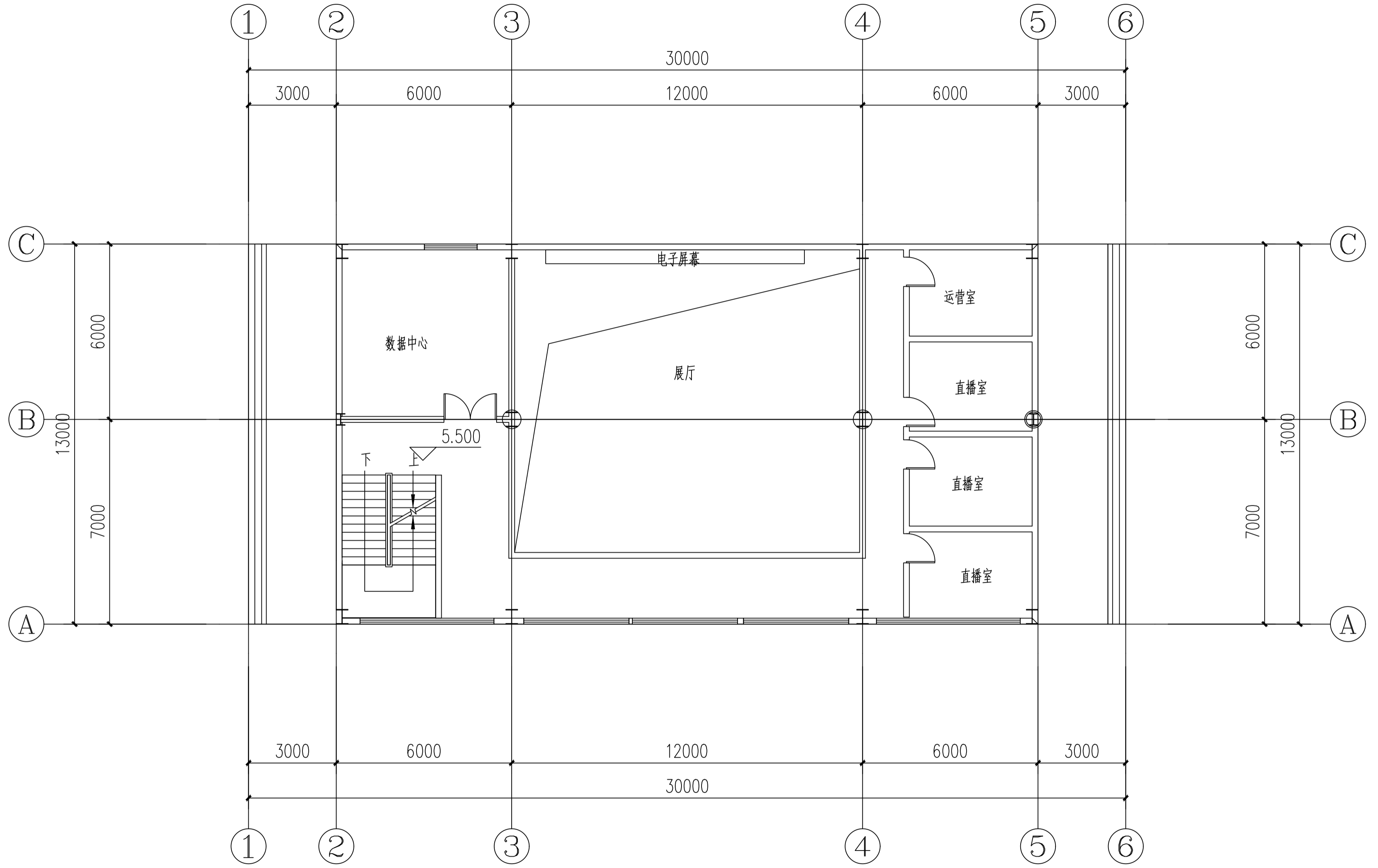
二层平面图 1:150
